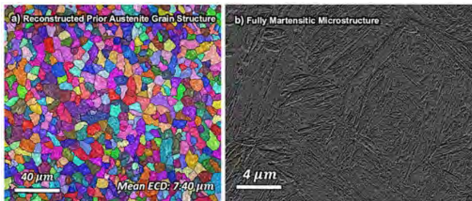
Kuva 5. a) rekonstruoitu austeniittinen raerakenne ennen induktiokarkaisua, ja b) lopullinen mikrorakenne induktiokarkaisun jälkeen (optimaaliset lämpökäsittelyparametrit, kuumnennus- ja jäähdytysnopeus 50 °C/s ja huippulämpötila 850 °C).
