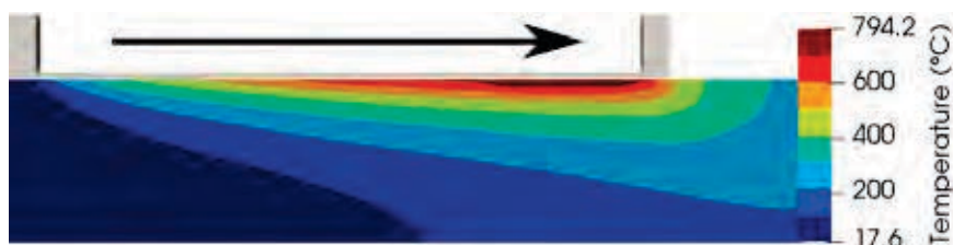
Kuva 15. Tuloksena saatava lämpötila induktiokelan alapuolella olevassa teräslevyssä. Nuoli osoittaa teräslevyn liikkumissuunnan.
