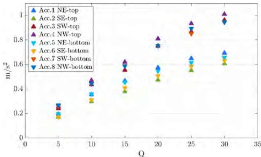
Kuva 10. Mitattu senkan seinämän värähtelykiihtyvyys ( \text{m/s}^2 ) kaasuhuuhteluvoimakkuuden ( \text{Nl/min} ) funktiona eri mittauspisteissä.
