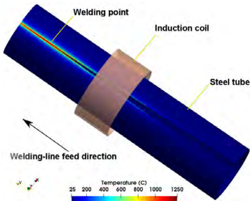
Kuva 1. Muovautuneen rainan reunojen ja hitsin muutosvyöhykkeen (HAZ) lämpötilajakauma.
