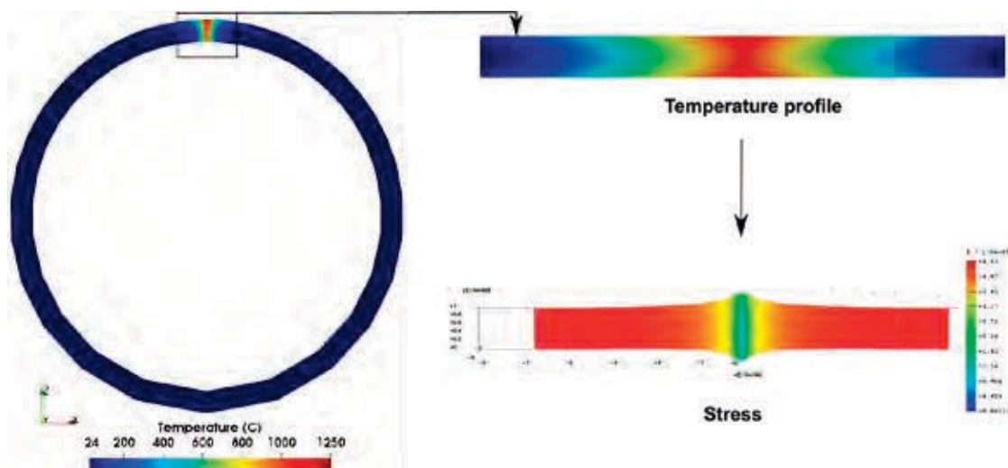
Kuva 2. Kaksiulotteinen hitsausliitoksen HAZ-alue hitsauspisteessä: lämpötilaprofiili ja jännitys.
