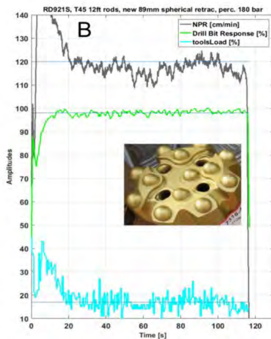
Kuva 3. Oikean porakruunun valinnalla kulloiseenkin kiviolosuhteeseen on suuri merkitys porauksen optimoinnissa. Esimerkissä on graniittisessa gneississä (DRI 47, UCS 110 MPa) tapahtunut poraus eri kruunuvaihtoehtoilla. Diagrammissa A poraus on suoritettu ballistisella kruunulla ja diagrammissa B pyöreänastaisella kruunulla. NPR eli tunkeumanopeus (cm/min) on saatu kasvatetuksi lähes 10 % valitsemalla olosuhteeseen sopiva kruunu. Kruunu-kivi -@kontakti (RockPulsen Drill Bit Response-mittarin perusteella) on saatu noin 8 % paremmaksi, ja kalustoa kuluttavien iskun paluuheijastuksien määrää (RockPulsen Tools Load-mittarin perusteella) on vähennetty noin 55 %.
