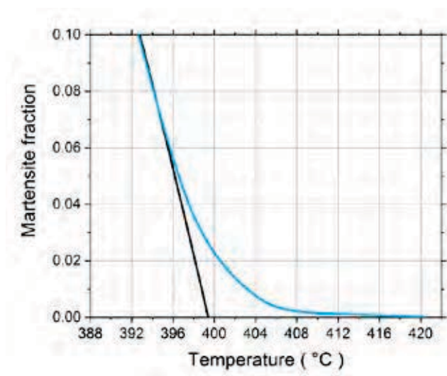
Kuva 16. Martensiitin kokonaistilavuusosuus lämpötilan funktiona. Sininen viiva perustuu sataan mitattuun paikalliseen koostumukseen ja musta viiva pohjautuu keskimääräiseen koostumukseen.
