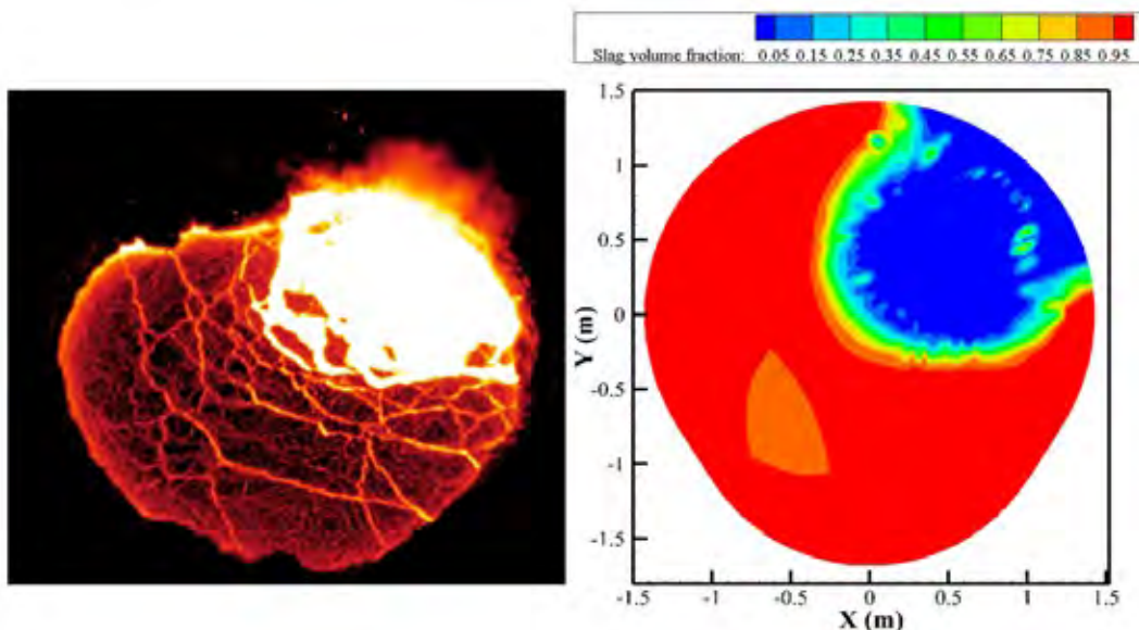
Kuva 9. Kuvattu (vasen) ja simuloitu (oikea) avoimen silmäkkeen koko 150 tonnin terässenkassa (400 Nl/min kaasuhuuttelu, 40 cm kuonakerros). [10]
