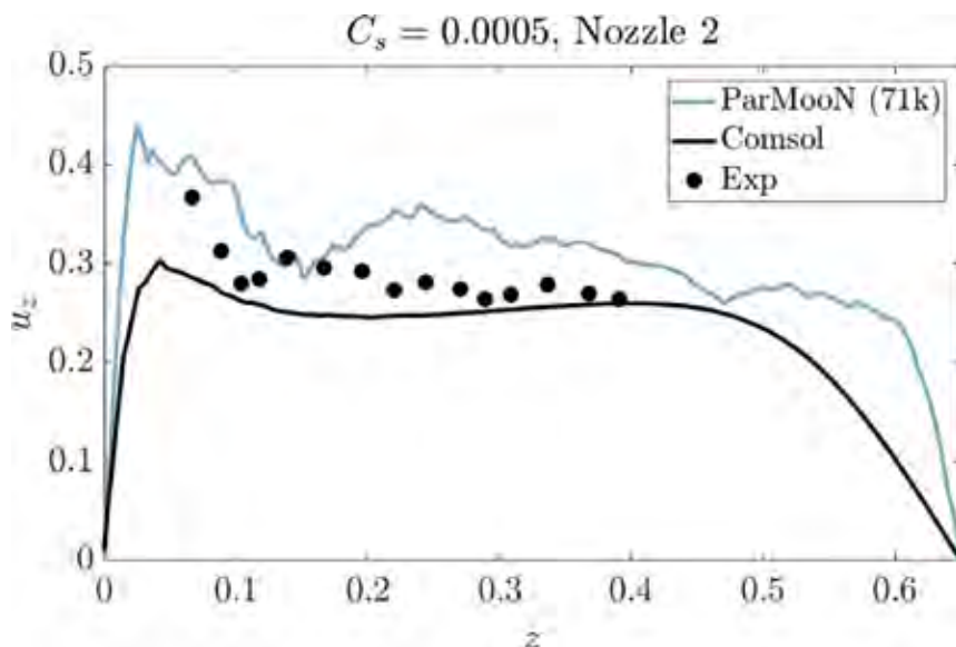
Kuva 11. Laskettu ja fysikaalisesta mallista mitattu pystysuuntainen kaasun nopeus ( \text{m/s} ) kaasupatsaan keskiliinjalla vesipatjan korkeuden ( \text{m} ) funktiona.
