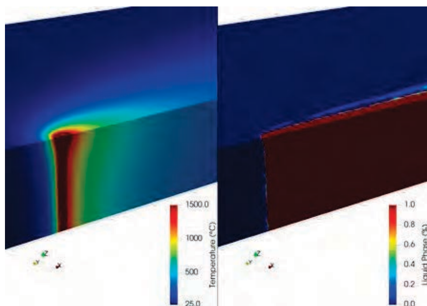
Kuva 13. Lämpötilajakauma ja polttoleikkauksen synnyttämän sulan teräksen faasisuus.
