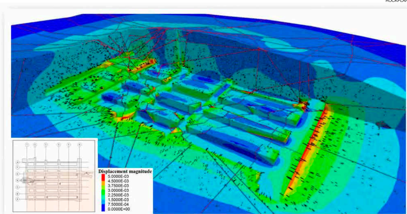
Kuva 5. Mallinnettujen kalliosiirtymien jakautuminen louhittavissa tiloissa. Siirtymät ovat millimetrituokkaa.
